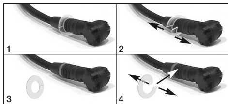
Fig. 3 : Remplacement de la bague collectrice
