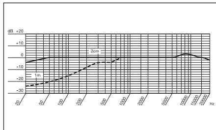
Frequenzkurve
