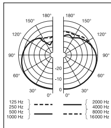
Polardiagramm
