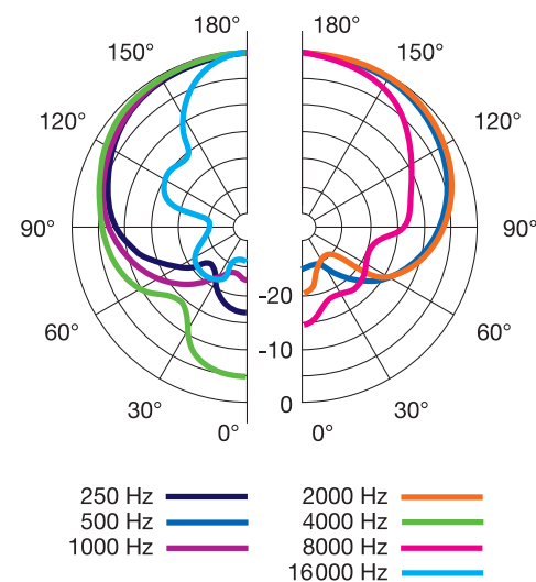
Polardiagramm D12 VR
